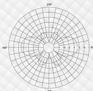
Polarização Horizontal
