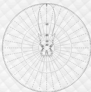
Polarização Horizontal
