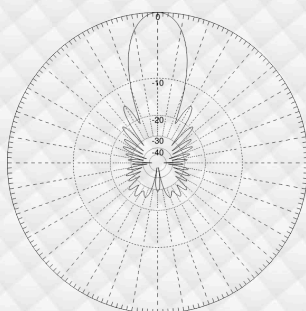
Polarização Vertical
