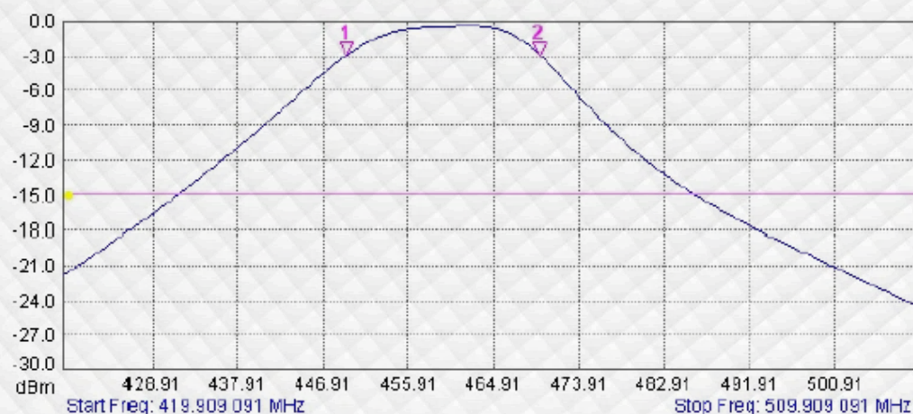
Transmission Measurement Data MINI FILTRO UHF 450~470MHz
