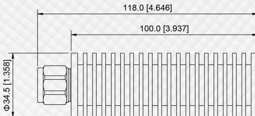
DESENHO MECÂNICO
