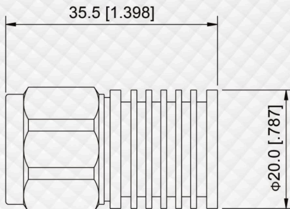
DESENHO MECÂNICO
