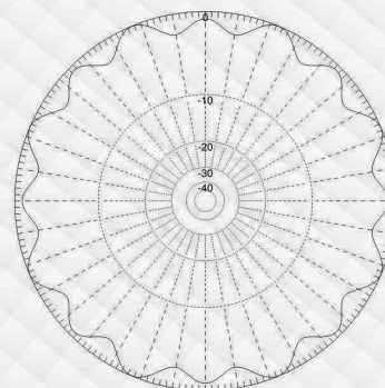
POLARIZAÇÃO HORIZONTAL
