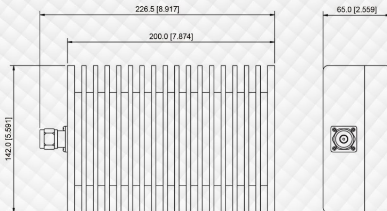
DESENHO MECÂNICO
