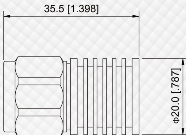
DESENHO MECÂNICO
