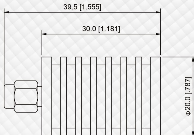
DESENHO MECÂNICO
