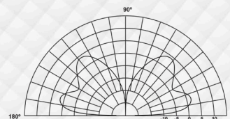
Polarización vertical
