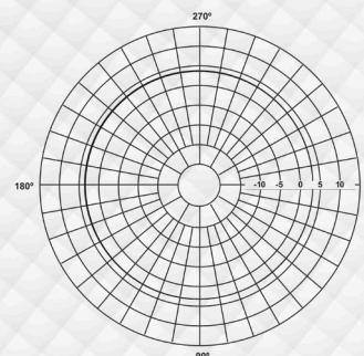
Polarización horizontal
