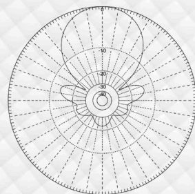
POLARIZAÇÃO VERTICAL
