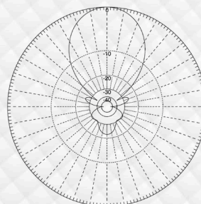
POLARIZAÇÃO HORIZONTAL
