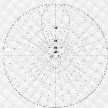
Polarización Horizontal
