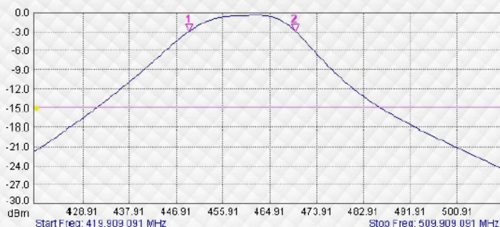
Transmission Measurement Data MINI FILTRO UHF 450~470MHz
