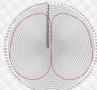
Polarización Vertical
