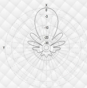
Polarização Vertical
