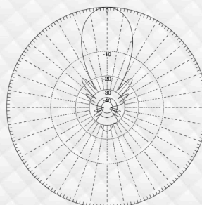
Polarización Horizontal
