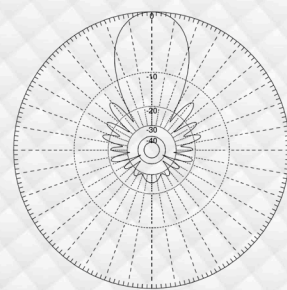
Polarización Vertical
