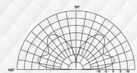
Polarização vertical
