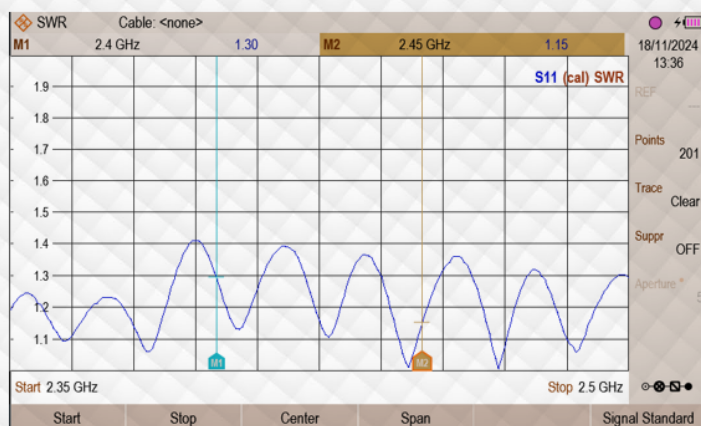
Polarização horizontal
