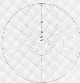
Polarização Vertical
